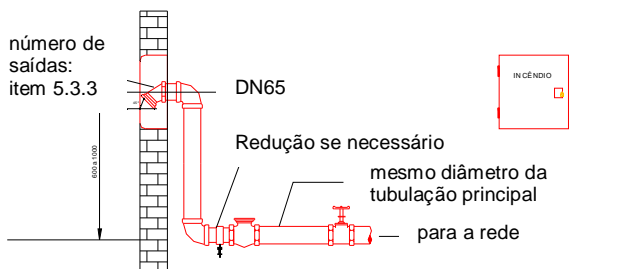
Figura 1 – Dispositivo de recalque tipo coluna
