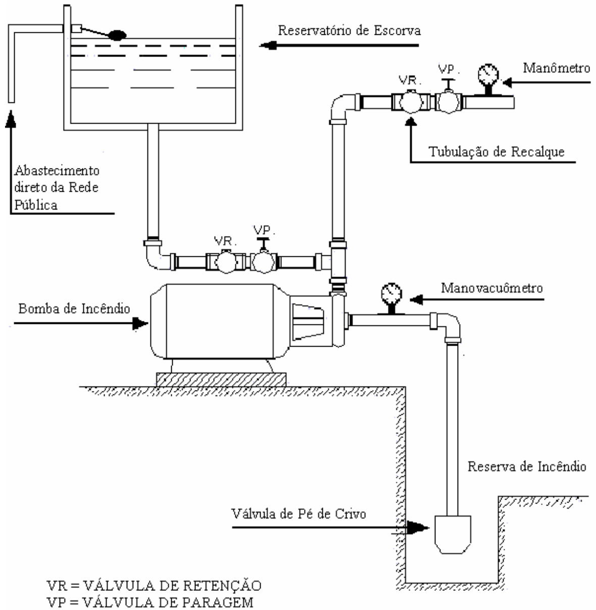
Figura C.3 – Exemplo de afogamento de bomba de incêndio
