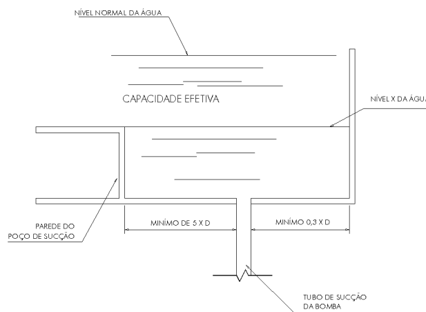
Figura B.2 - Tomada lateral de sucção para bomba principal
