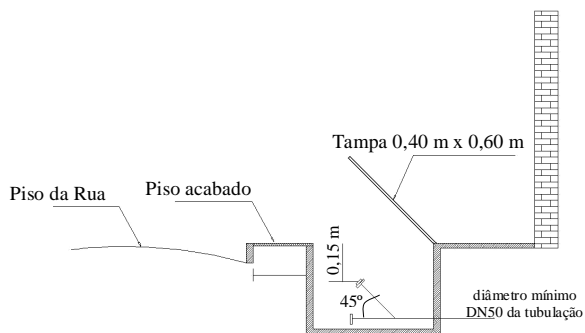
Figura 2 – Dispositivo de recalque no passeio público
