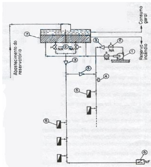
Figura C.5 - Esquema de instalação de bomba de reforço abastecendo os pontos de hidrantes ou mangotinhos mais desfavoráveis considerados no cálculo, por uma só prumada,.
