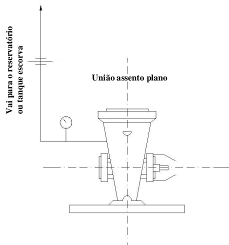
Figura C.6 – Arrefecimento da bomba principal elétrica
